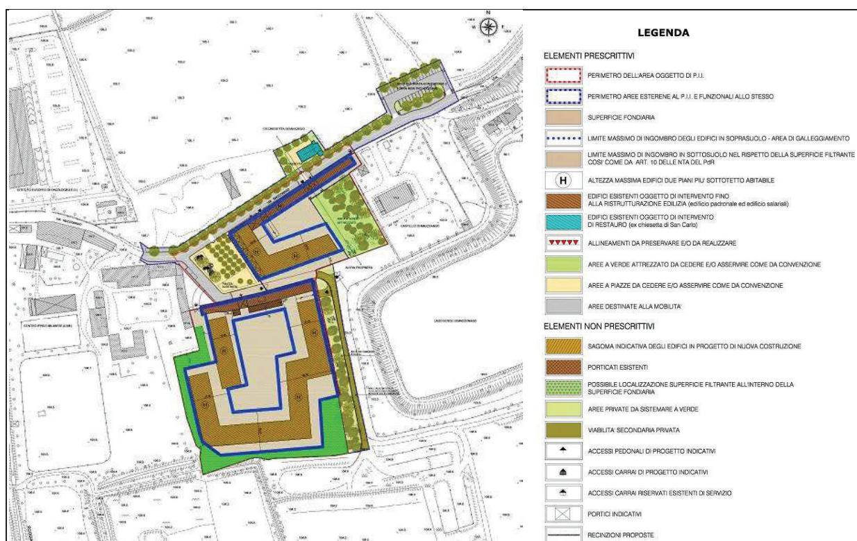
Planivolumetrico prescrittivo di progetto
